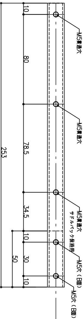
角パイプ 15×15×1.5 部品図
